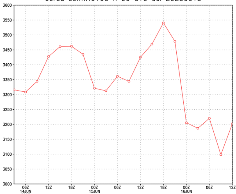
Zero termico Ancona corsa ecmwf0100 h 00 UTC del 20230613
